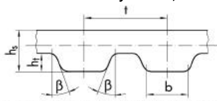
Aufbau: Polyurethan mit Stahlzugstrang
