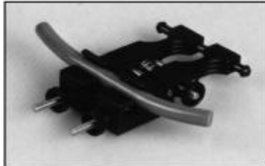
Führungszange B 3
